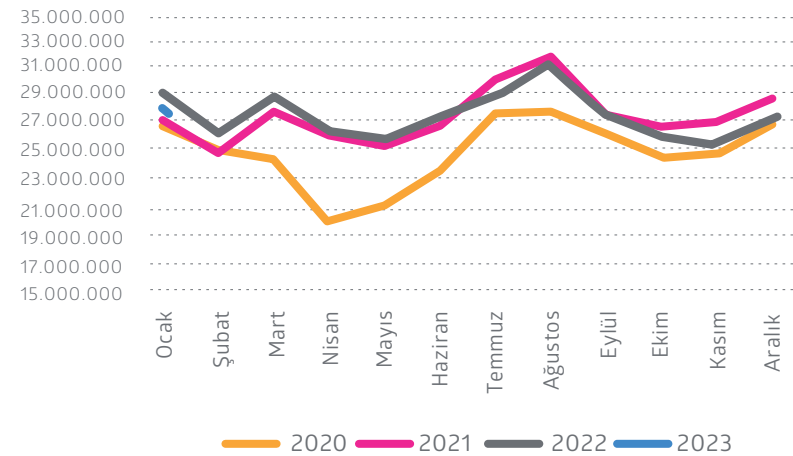
2020-2023 Türkiye Toplam Tüketimi (MWh)
