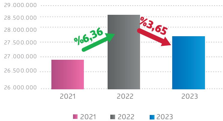
2021-2023 Türkiye Toplam Tüketimi (MWh) (01 Ocak-31 Ocak)
